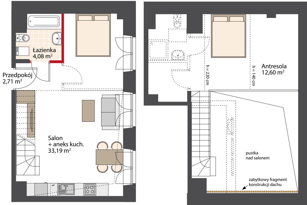
1 PIĘTRO
